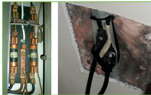
Dérivations électriques
